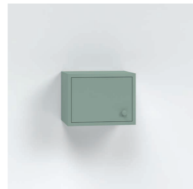
OM400D Bredd: 400 mm. Djup: 315 mm. Höjd: 300 mm.
