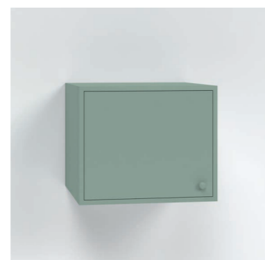
HM500 Bredd: 600 mm. Djup: 600 mm. Höjd: 500 mm.
